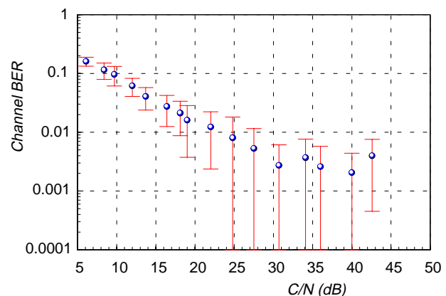
b) RURAL1 channel, 50 km/h
